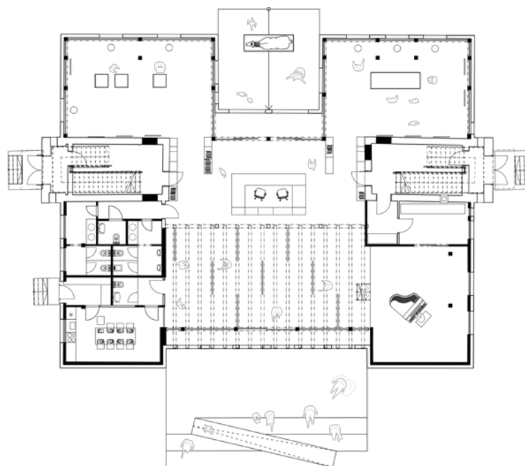
↑ Pôdorys 1. NP.
